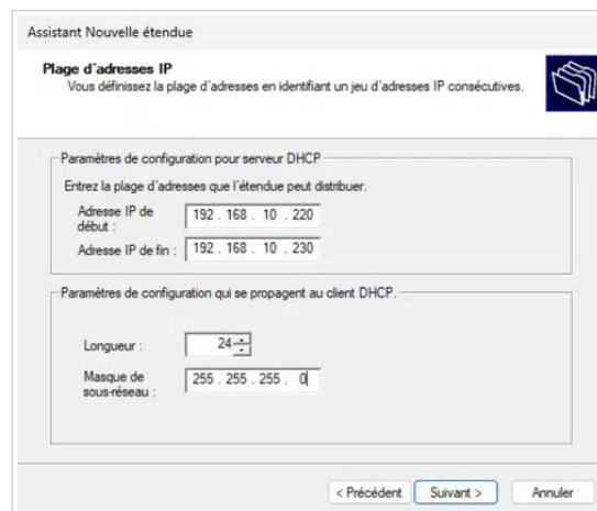
Définition de la plage d'adresses IP
