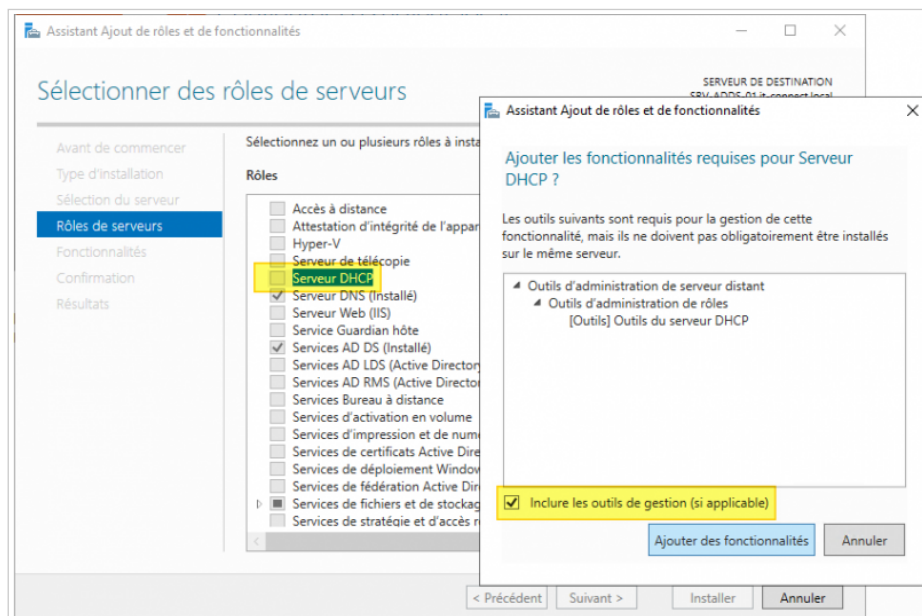
Sélection du rôle Serveur DHCP
