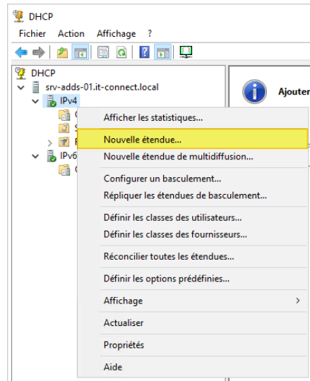
Console DHCP — Nouvelle étendue sur IPv4
